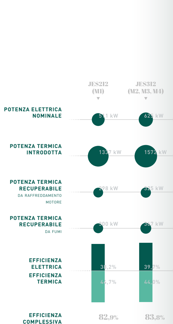
FIG 3.10 Impianti di cogenerazione dal biogas
