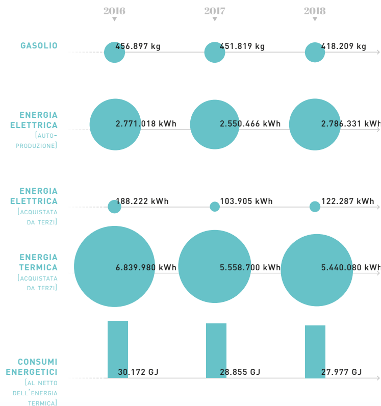
FIG 4.5 Consumi energetici di Belvedere
