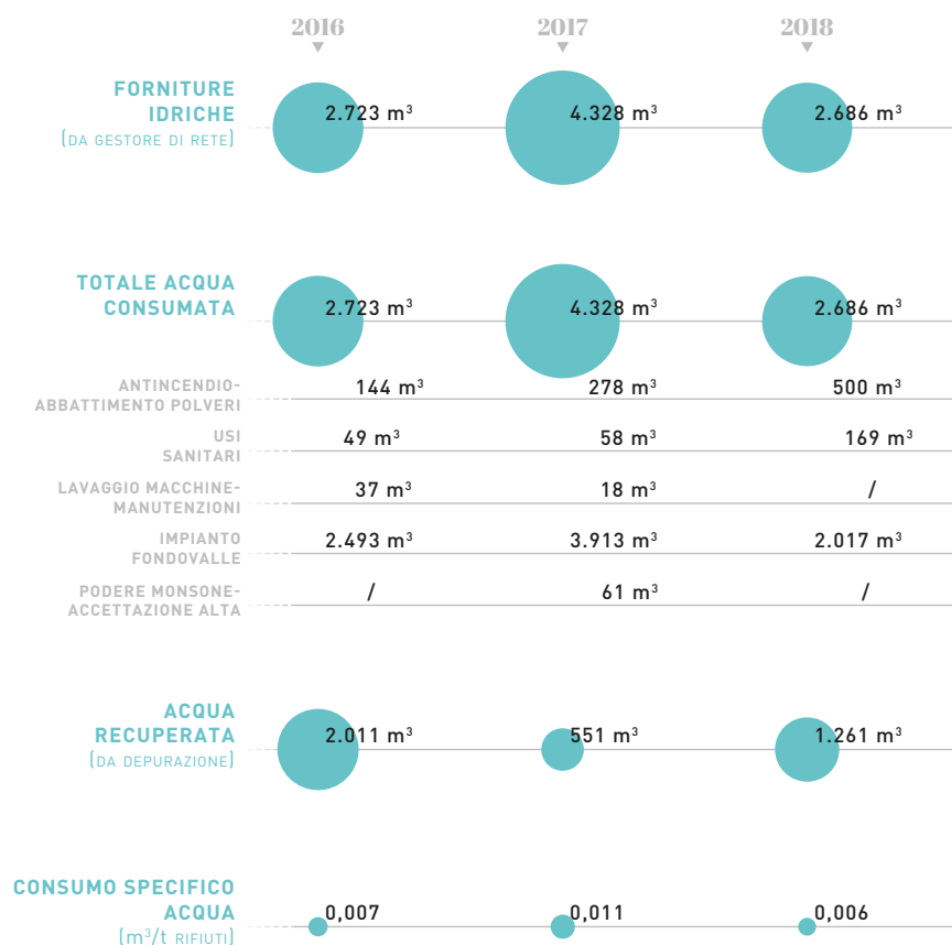
FIG 4.17 Acqua prelevata, consumata, recuperata
