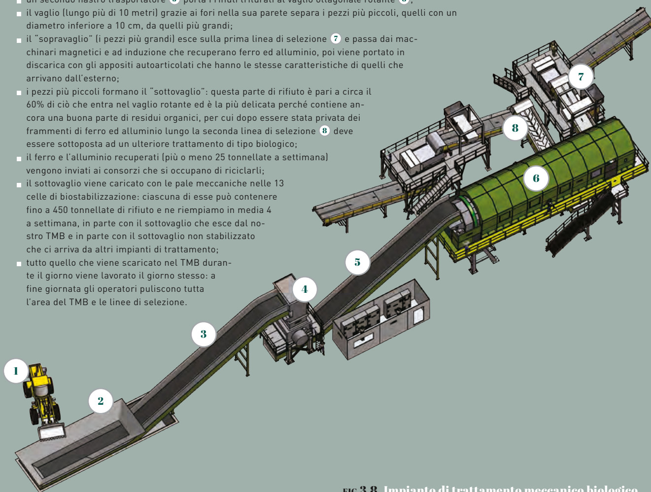
FIG 3.8 Impianto di trattamento meccanico biologico
