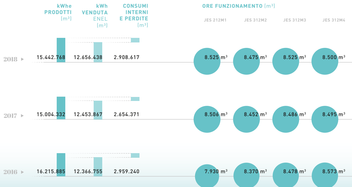
FIG 4.8 Produzione di energia elettrica dall'impianto di cogenerazione
