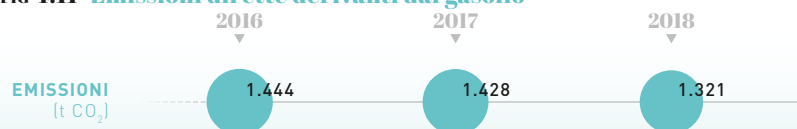
FIG 4.11 Emissioni dirette derivanti dal gasolio*
